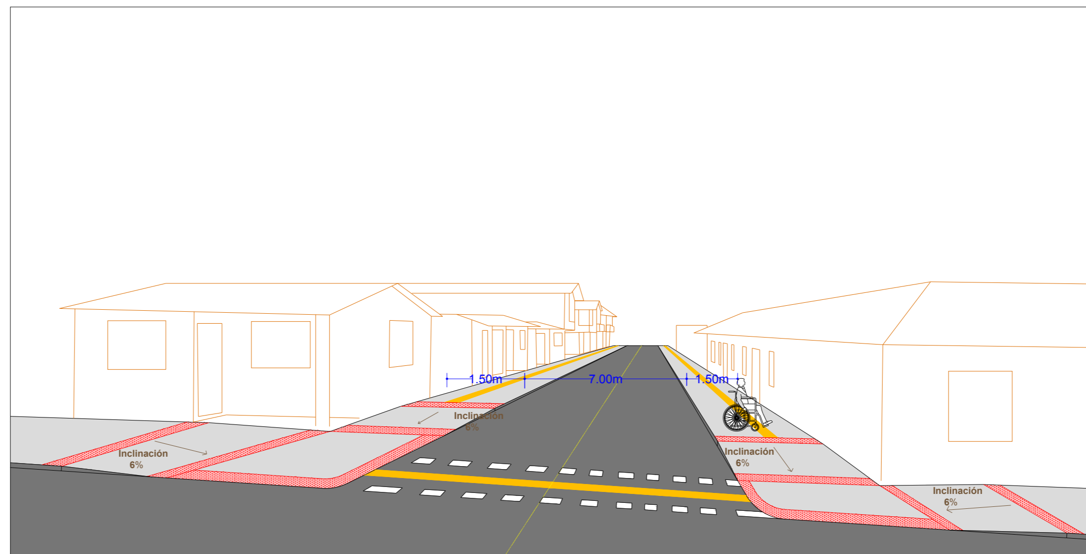
Corte S-S'
