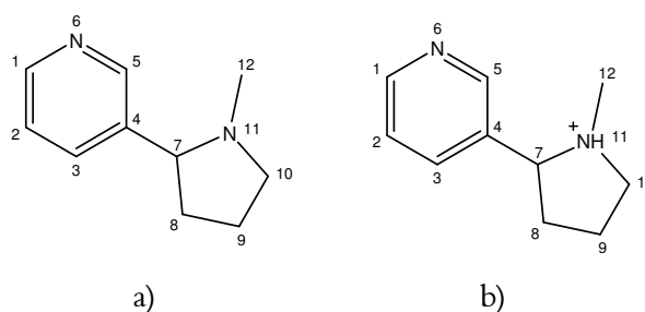
Figura 1. Estructuras bi-dimensionales de la molécula de nicotina (N); (a) no protonada, (b) monoprotónada ( \text{NH}^+ ).
