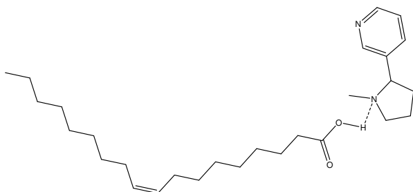
Figura 2. Estructura bidimensional de ácido oleico-nicotina. La interacción de enlace de hidrógeno entre el grupo carboxílico de la molécula de ácido oleico y el grupo pirrolidínico de la molécula de nicotina está indicada con la línea punteada.
