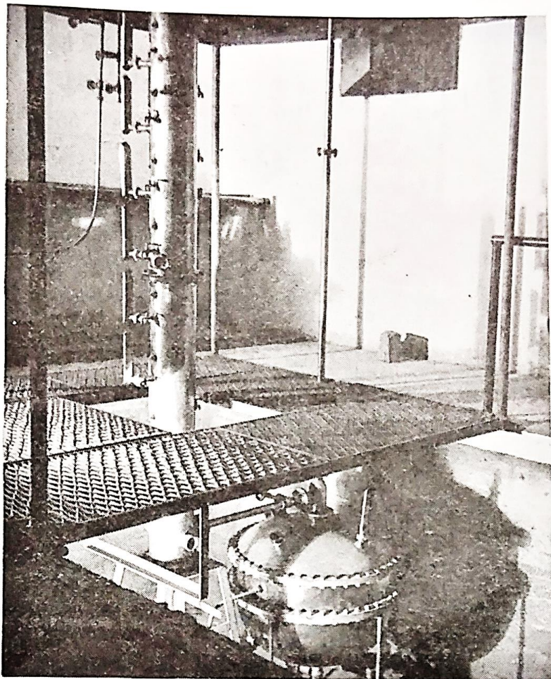
Laboratorio de Operaciones Unitarias. Torre de destilación de platos y cápsulas, con termómetro y llaves para tomar muestras de los distintos platos.
