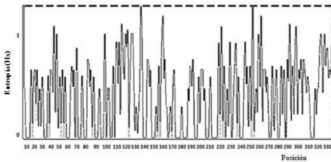
Figura 3. Entropía H(x) en la secuencia de nucleótidos parcial del gen citocromo b de L. trinidadensis , L. panamensis , L. c. cayennensis , L. dubitans , L. gomezi , L. rangelifana y L. evansi .
