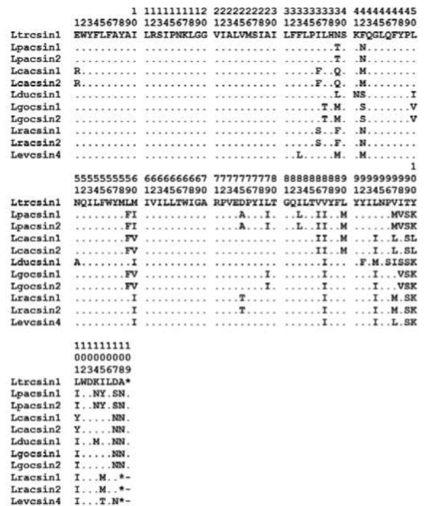
Figura 2. Alineamiento de secuencias aminoácídicas del dominio carboxilo terminal de la proteína citocromo b de L. trinidadensis (Ltrcsin1), L. panamensis (Lpacsin1, Lpacsin2), L. c. cayennensis (Lcacsin1, Lcacsin2), L. dubitans (Lducsin1) y L. gomezi (Lgocsin1, Lgocsin2), L. rangelifiana (Lracsin1, Lracsin2) y L. evansi (Levcsin4). Los aminoácidos se representan con su código universal de una letra, las homologías con puntos, los eventos indel (inserción-delección) con guiones y los codones de parada con asteriscos.
