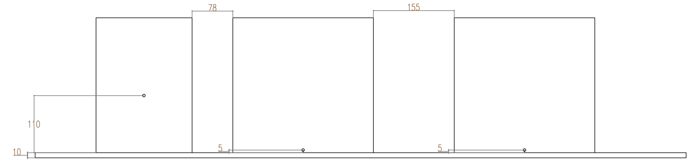
PLANTA DE POTABILIZACIÓN SIN TUBERÍAS VISTA LATERAL DERECHA
