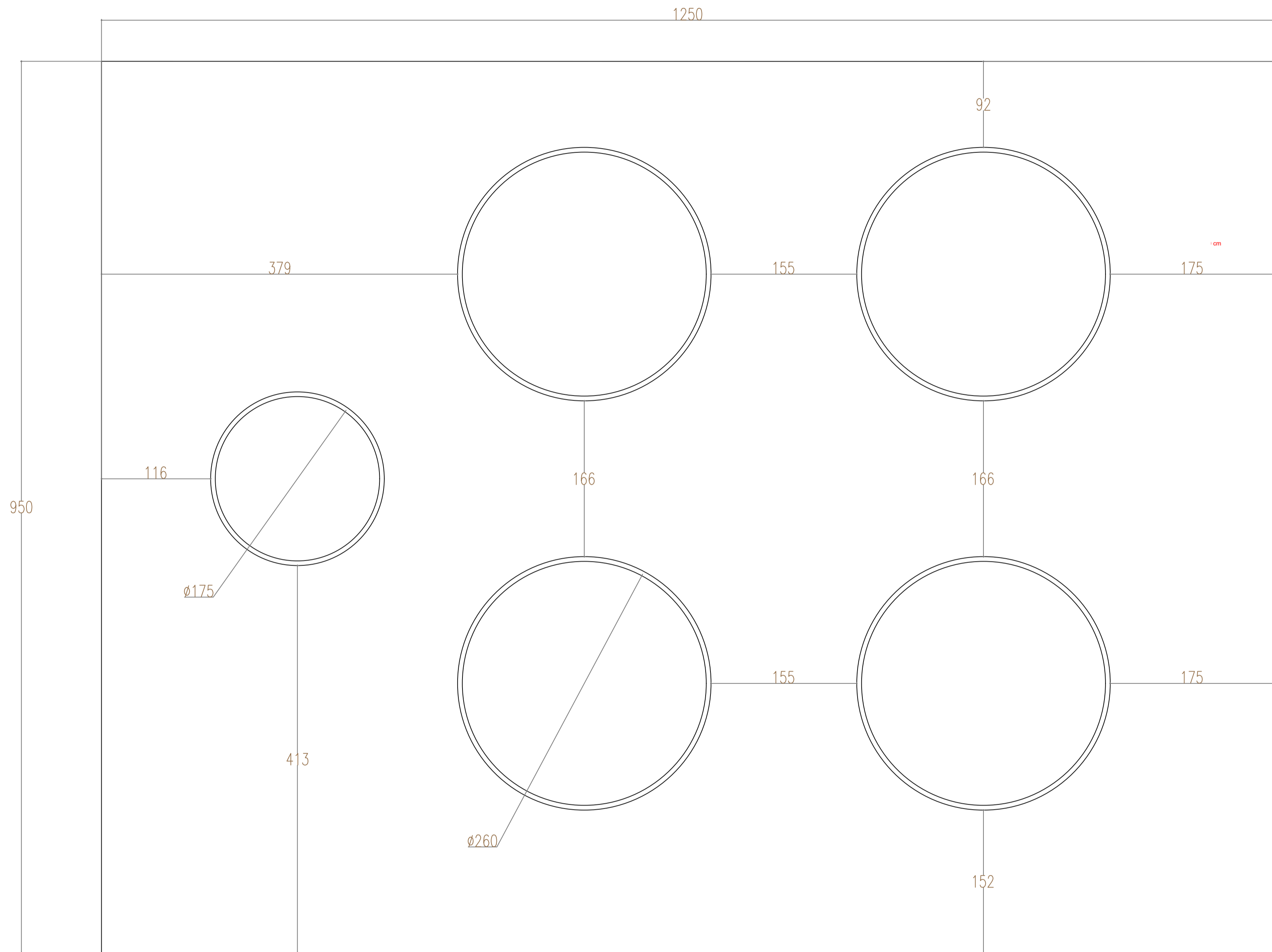
PLANTA DE POTABILIZACIÓN SIN TUBERÍAS VISTA EN PLANTA
