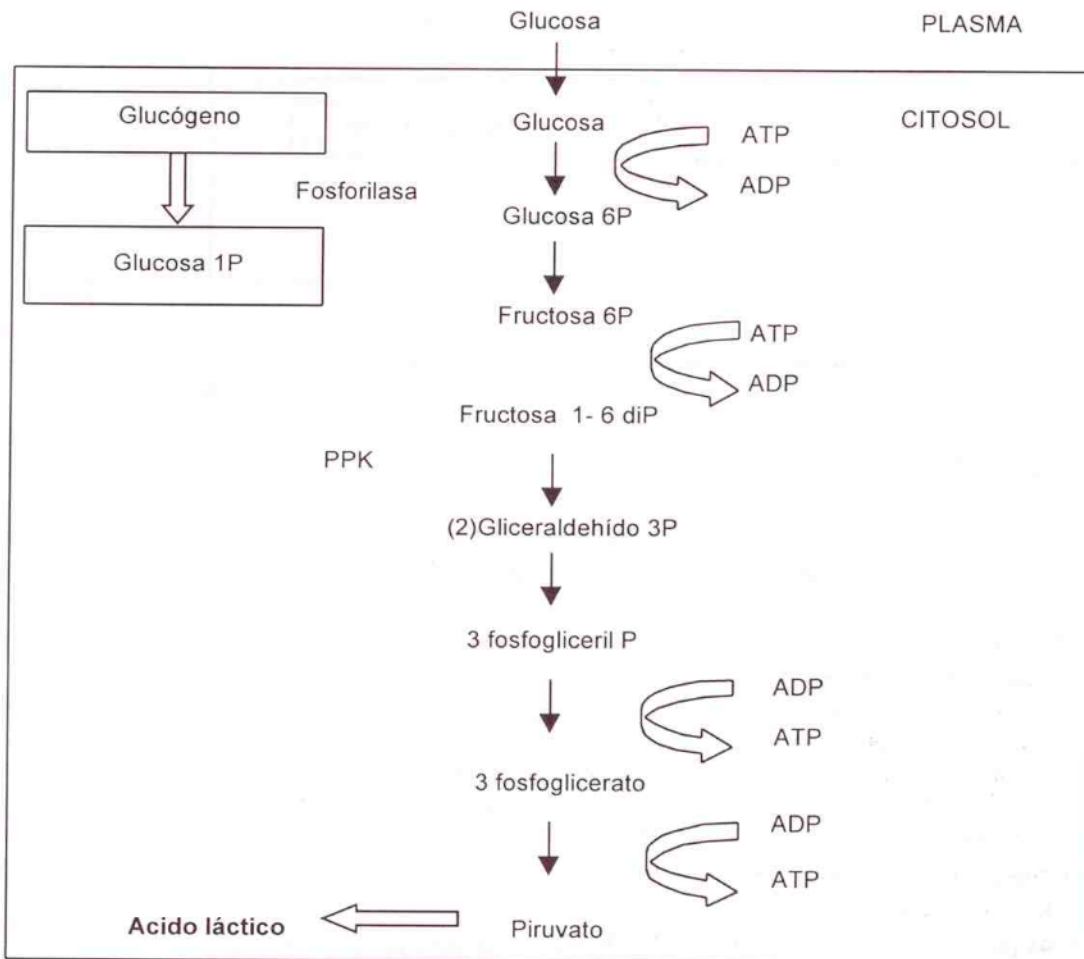
Figura 2. Esquema general del metabolismo anaeróbico láctico en la célula muscular
