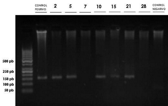
Figura 1. Electroforesis en gel de agarosa B.P.F. al 3% en 7 muestras de amplificadas para SRY de sangre de terneras nacidas por parto múltiple heterosexual en Colombia.
