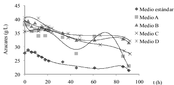
Figura 2 Efecto del reemplazo de la fuente de carbono sobre el consumo de azúcares
