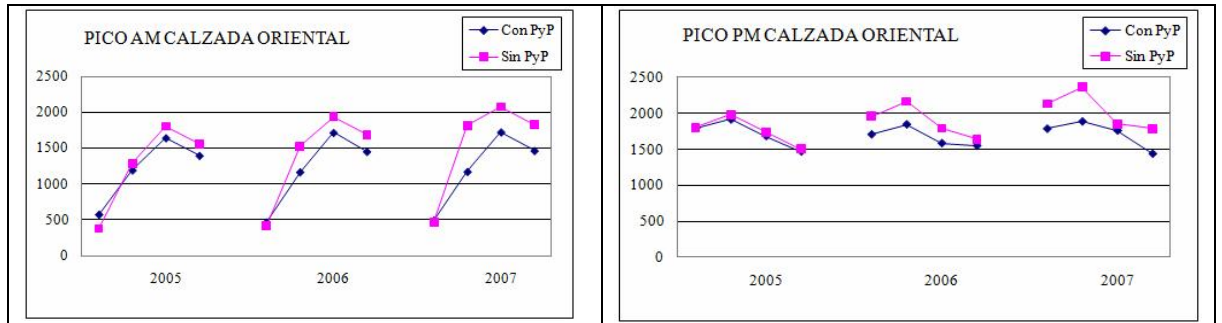
Figura 4. Volúmenes vehiculares con y sin Pico y Placa en horas de restricción. Estación Politécnico Figure 4. Vehicle volumes with and without restriction in peak hours. Station: Politécnico
