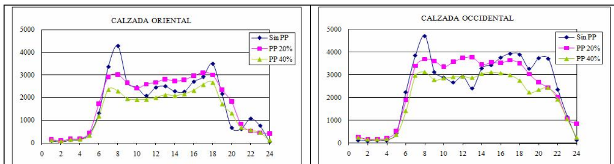
Figura 5. Volúmenes horarios sin Pico y Placa y con Pico y Placa del 20 y 40%. Estación: Autopista-Av. 33 Figure 5. Hourly volumes without restriction and with 20% and 40% restriction. Station: Autopista-Av. 33
