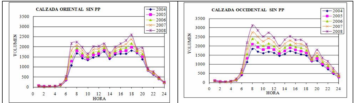
Figura 3. Volumen horario sin Pico y Placa. Estación: Politécnico Figure 3. Hourly Volumes without restriction. Station: Politécnico
