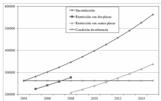
Figura 6. Evolución temporal del volumen vehicular sin Pico y Placa y con Pico y Placa del 20 y 40% Figure 6. Vehicular volume temporal evolution without restriction and with 20% and 40% restriction
