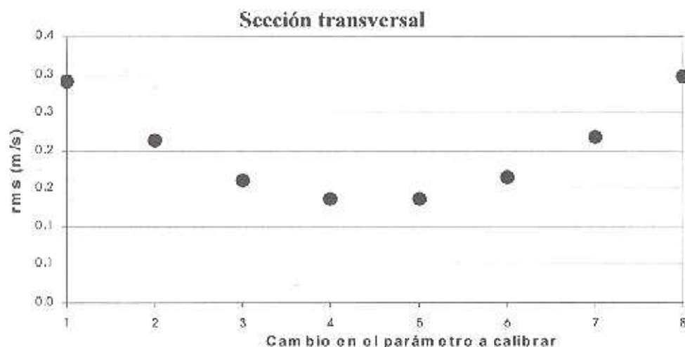
FIGURA 1. Análisis del estadístico "rms" en una sección transversal
