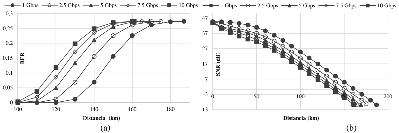
Figura 9. Curvas de lectura del código QR obtenido a la salida del receptor, aplicando PDI. (a) Relación BER vs Distancia y (b) Relación SNR vs Distancia. Fuente: Los autores.
