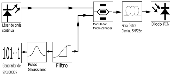
Figura 3. Sistema de comunicación a través de fibra óptica, diseñado con el software VPI photonics. Fuente: Los autores.
