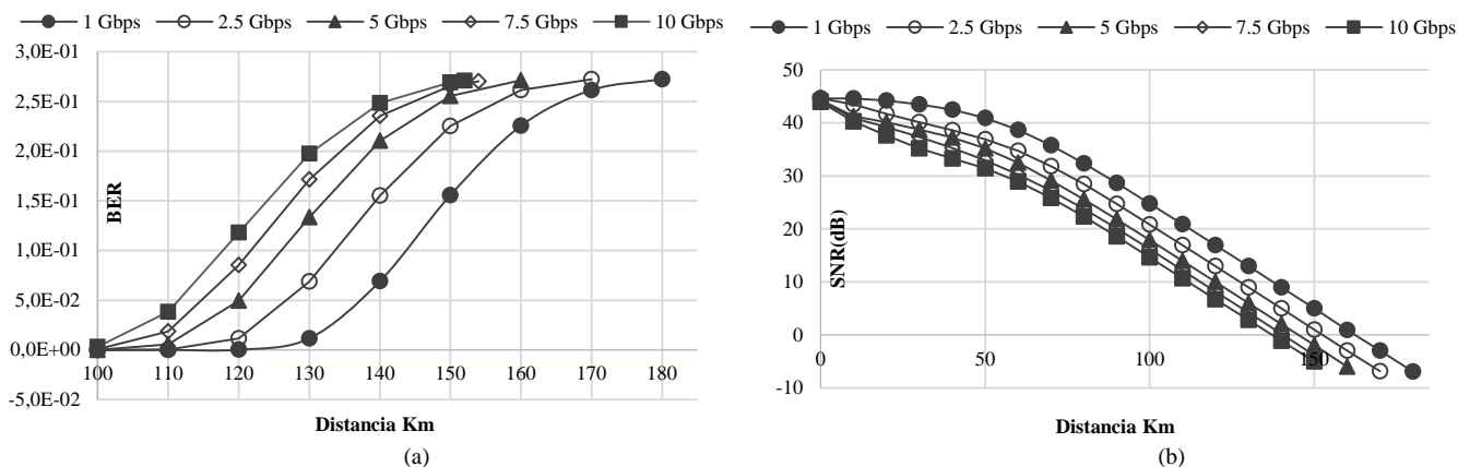
Figura 5. Curvas de lectura del código QR obtenido a la salida del receptor, con Smartphone. (a) Relación BER vs Distancia y (b) relación SNR vs Distancia. Fuente: Los autores.
