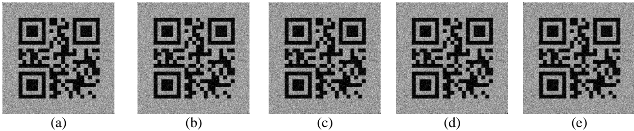
Figura 8. Códigos QR leídos vía Web (distancia crítica). (a) Tasa de transmisión 1 Gbps, distancia máxima 145 Km. (b) Tasa de transmisión 2,5 Gbps, distancia máxima 135 Km. (c) Tasa de transmisión 5 Gbps, distancia máxima 128 Km. (d) Tasa de transmisión 7,5 Gbps, distancia máxima 123 Km. (e) Tasa de transmisión 10 Gbps, distancia máxima 120 Km. Fuente: Los autores.
