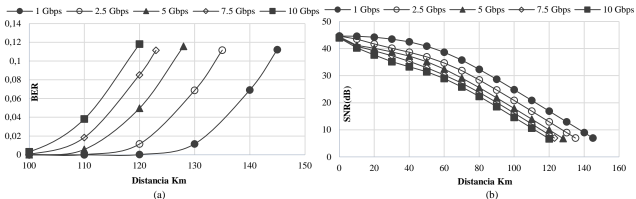
Figura 7. Curvas de lectura del código QR obtenido a la salida del receptor, vía web. (a) Relación BER vs Distancia y (b) Relación SNR vs Distancia. Fuente: Los autores.
