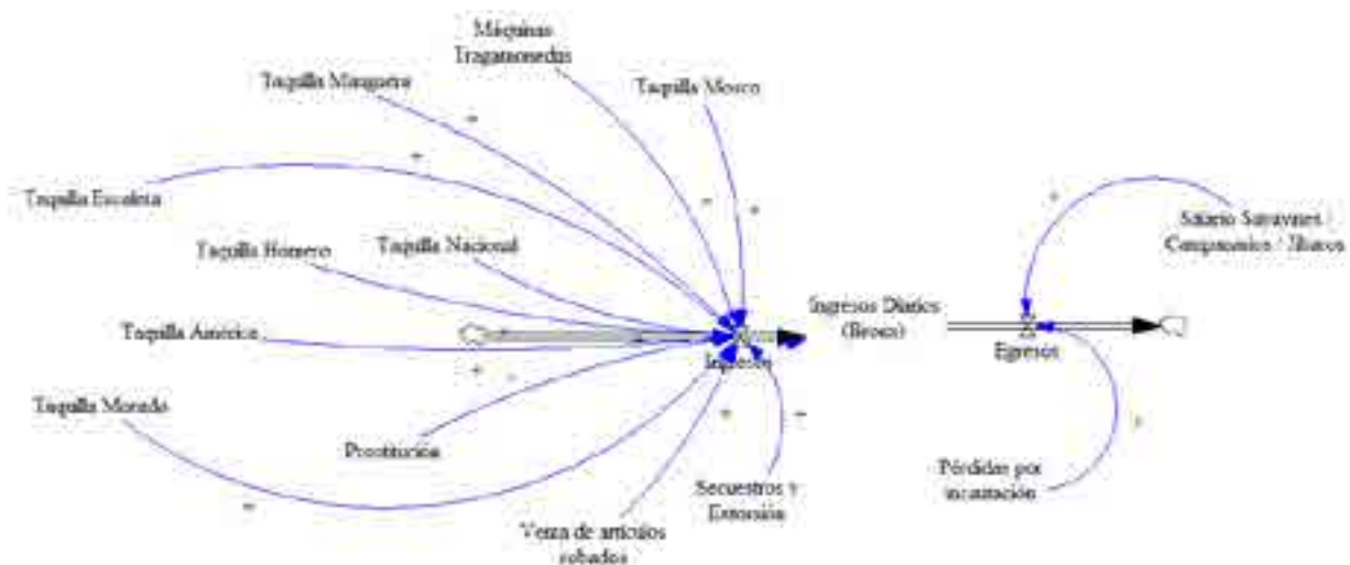
Figura 3. Diagrama causal
