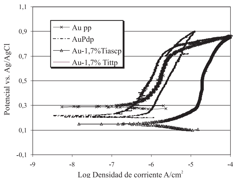
Figura 5 Curvas de segunda polarización para las muestras de oro puro pasivada (Au p), la aleación Au-Pd-Ga-In pasivada (AuPd), Au-1,7% Ti “as cast” pasivada (Au -1,7% Ti asc) y Au-1,7% con 4 h de envejecimiento pasivada (Au -1,7% Ti ttp). Todas las polarizaciones se realizaron en solución de Ringer desaireada a 37 °C
