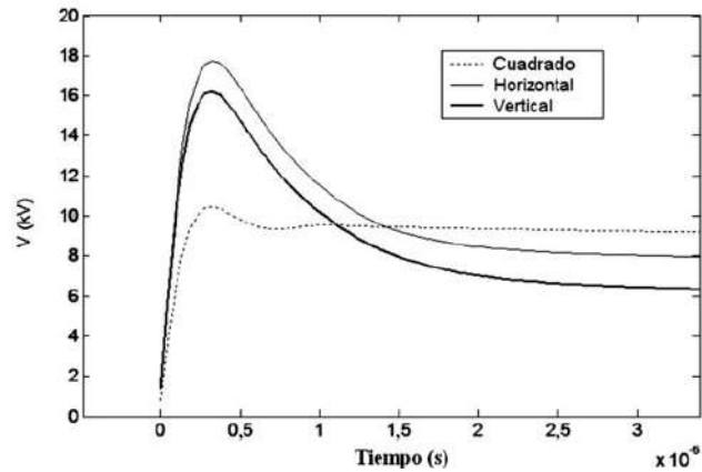
Figura 3 GPR transitorio para diferentes geometrías
