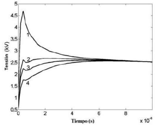
Figura 14 Sobretensiones en los puntos de observación
