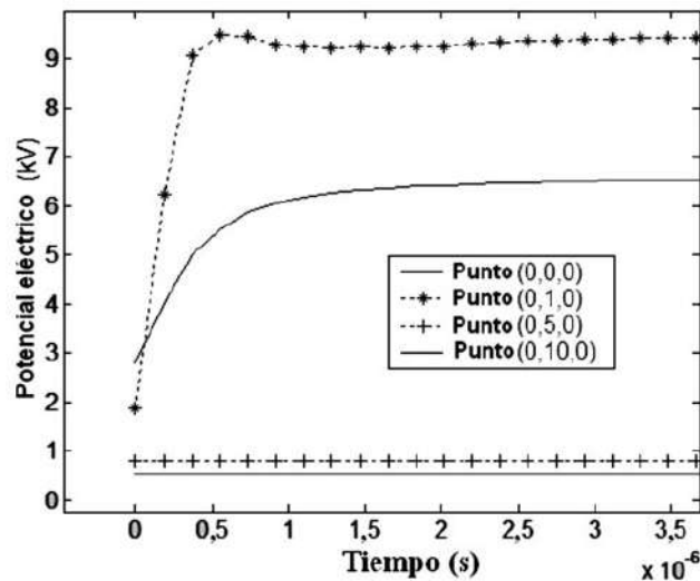
Figura 11 Tensiones de contacto y de paso sobre un contrapeso
