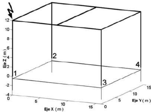
Figura 13 Sistema de protección contra rayos y ubicación de puntos de observación (1 a 4)
