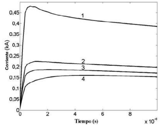
Figura 15 Corrientes en los puntos de observación
