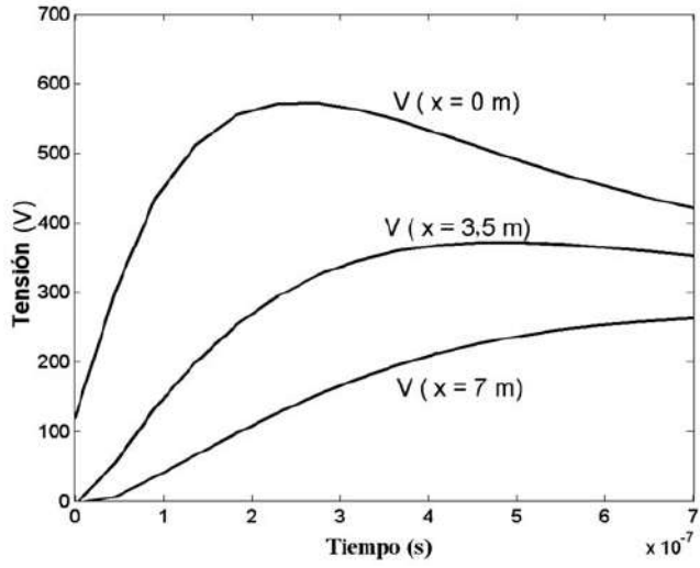
Figura 8 Efecto de la atenuación de las sobretensiones en un contrapeso de 15 m
