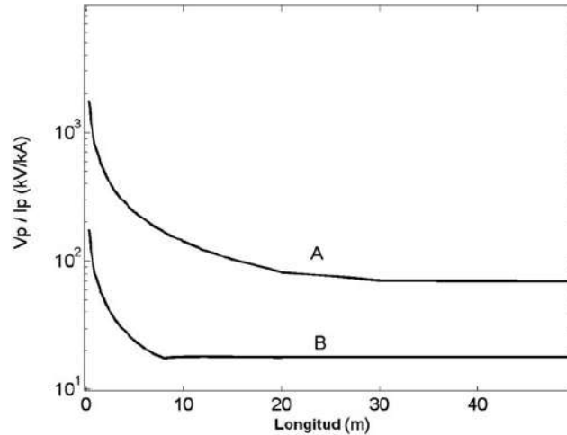
Figura 10 Impedancia impulso en función de la longitud de un contrapeso en dos suelos diferentes.
