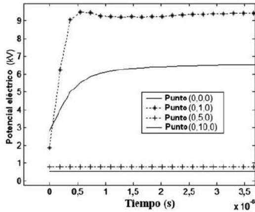
Figura 12 Potencial eléctrico en varios puntos de la superficie del suelo
