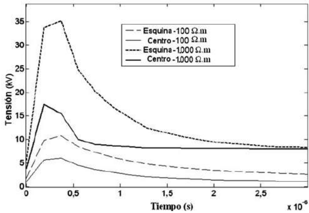
Figura 7 GPR transitorio para los casos de las figuras 5-6
