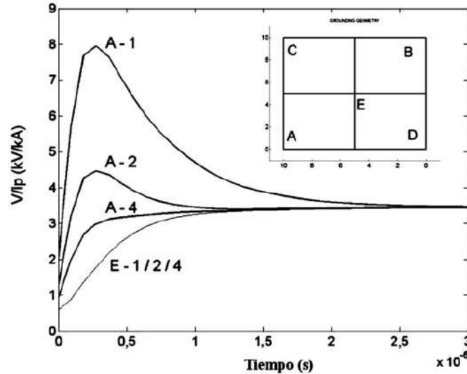
Figura 5 GPR transitorio normalizado para diversos puntos de inyección de corriente
