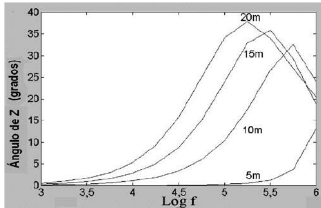
Figura 9 Variación de la impedancia con la frecuencia para diferentes longitudes de electrodos horizontales
