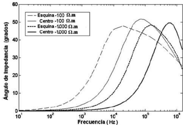
Figura 4 GPR transitorio para diversos frentes de onda
