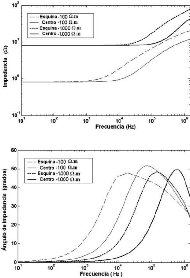
Figura 6 Influencia de \rho y \epsilon_r y de la localización del punto de inyección en la impedancia de PaT.
