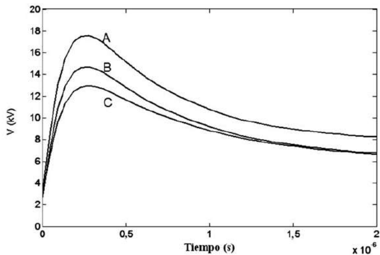
Figura 2 Influencia de la dependencia de los parámetros del suelo con la frecuencia en el máximo GPR transitorio
