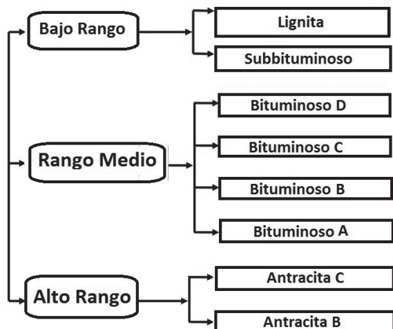
Figura 3. Clasificación de los carbones, según la norma ISO 11760-2005.
