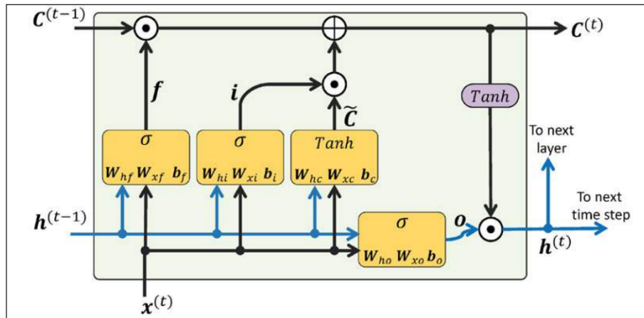
Figura 2.3: Estructura desmenuada de una celda LSTM [13].
