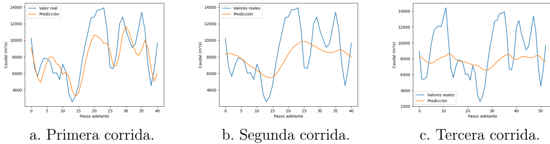
Figura 3.9: Comparación entre las diferentes corridas para las predicciones del modelo LSTM y los valores reales.
