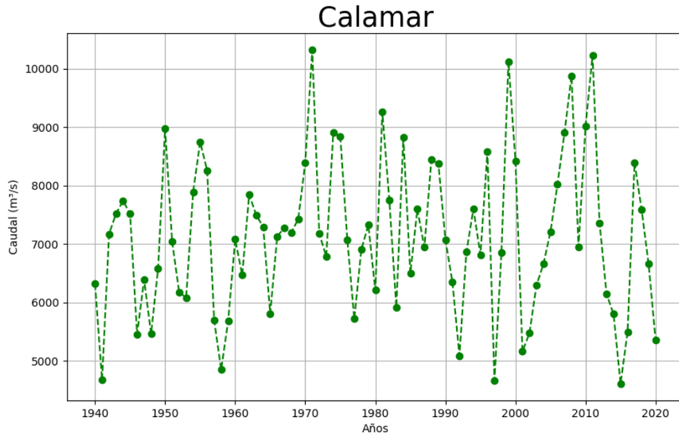
Figura 3.4: Histórico con el promedio anual del caudal de la estación hidrológica de Calamar.
