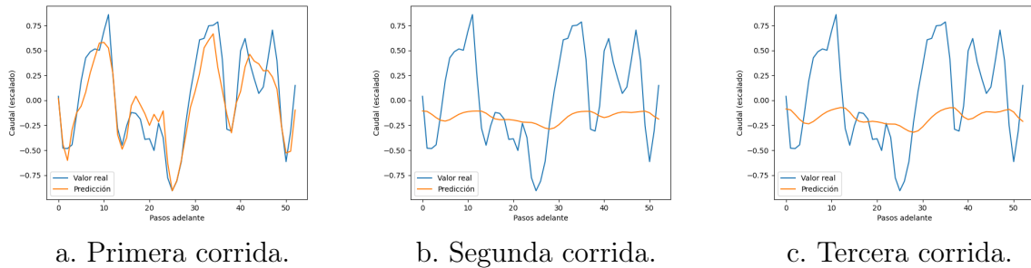
Figura 3.11: Comparación entre las diferentes corridas para las predicciones del modelo GRU y los valores reales.
