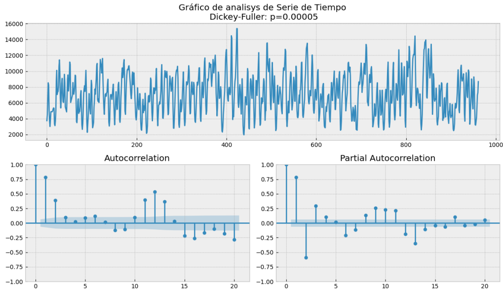
Figura 3.5: Gráfico de Autocorrelación y Autocorrelación Parcial.
