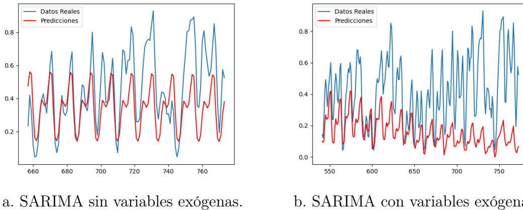
Figura 3.6: Predicciones con el modelo SARIMA.
