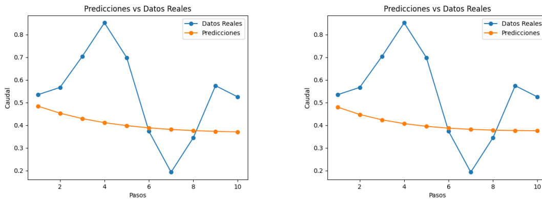
a. VAR con cuatro índices climáticos.
