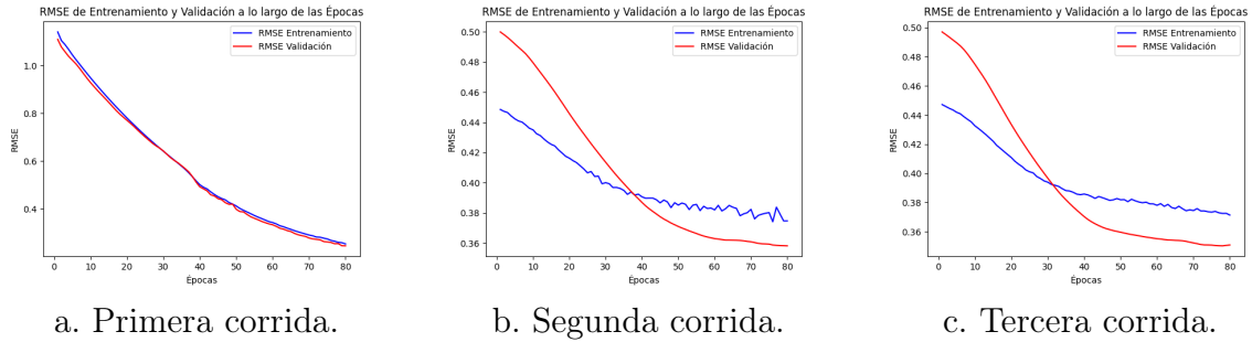
Figura 3.10: Comparación entre las diferentes corridas para el modelo GRU.
