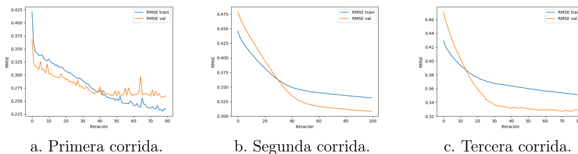
Figura 3.8: Comparación entre las diferentes corridas para el modelo LSTM.
