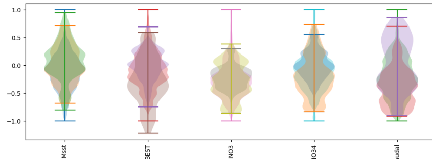
Figura 3.7: Diagrama de Violín para las series de tiempo.
