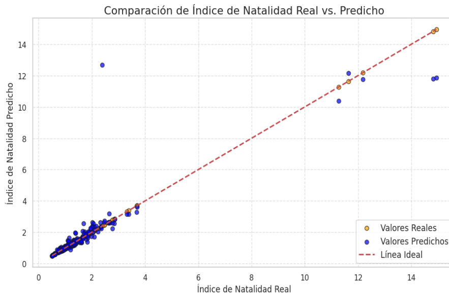
Figura 7. Gráfico de regresión: Índice de natalidad predicho vs real, utilizando XGBoost.
