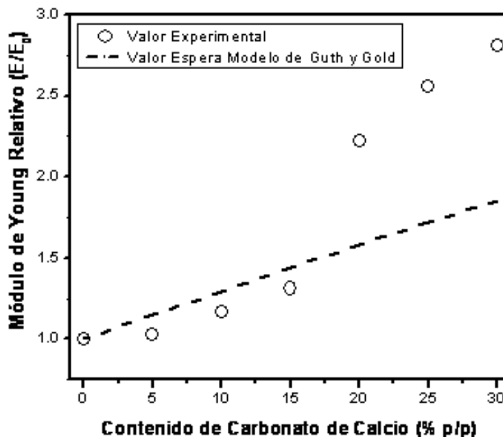
Figure 4. Valores de módulo elástico para cada una de las composiciones de carbonato de calcio y su ajuste al modelo de Guth y Gold.
