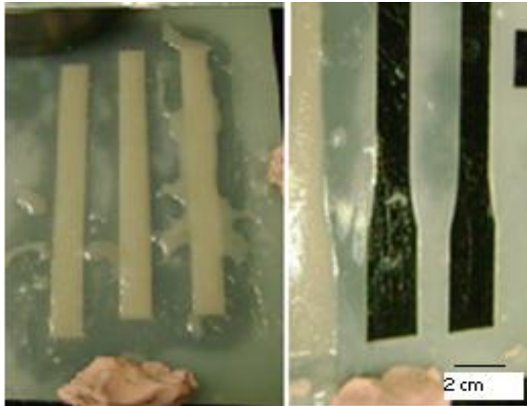
Figura 1. Fotografía de las probetas empleadas para HDT (izquierda) y resistencia a la tracción (derecha).
