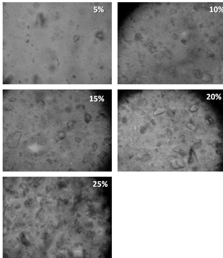
Figura 5. Micrografías ópticas de luz transmitida para diferentes composiciones de los materiales compuestos a 40x.
