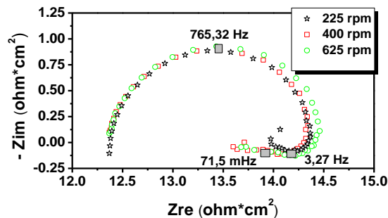
Figura 1. Resultados de impedancia durante el depósito de los recubrimientos de Ni a las diferentes velocidades de rotación.
