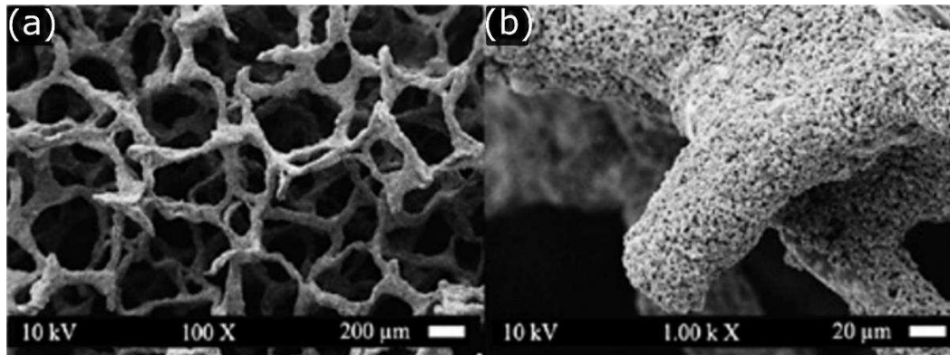
Figura 3. Scaffold de vidrio bioactivo recubierto con microesferas de PHBV a) 100 X; b) 1000 X [52].
