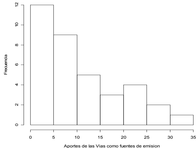
Figura 1. Distribución de frecuencias de contribución de las vías Figure 1. Road Contribution frequencies distribution
