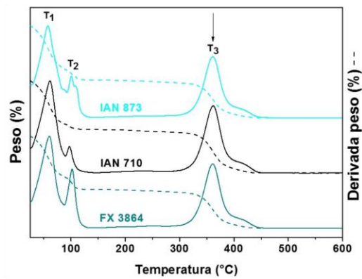
Figura 2. Termogravimetría de las muestras evaluadas.
