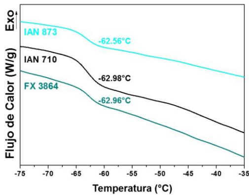
Figura 1. Tg de las muestras evaluadas.
