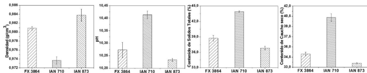
Figura 4. Análisis fisicoquímico usando la norma técnica ASTM D1076.
