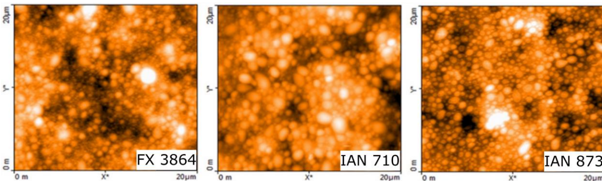
Figura 3. Morfología de las partículas de látex. Modo topográfico en AFM
