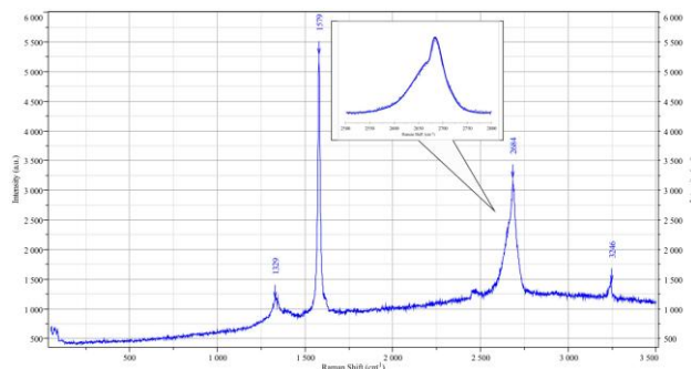
Figura 5. Espectro Raman del FLG-RG con pocos defectos de borde
