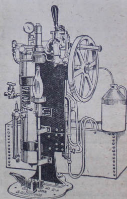
Máquina "B" de FLUGEL con llenador para Botellas con Tapones de Corón.
